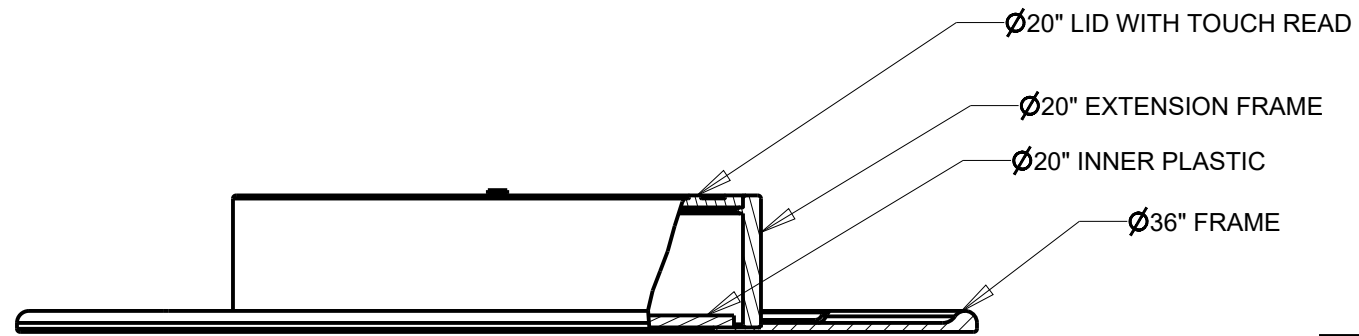
SECTION A-A
