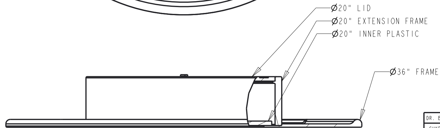
SECTION A-A
