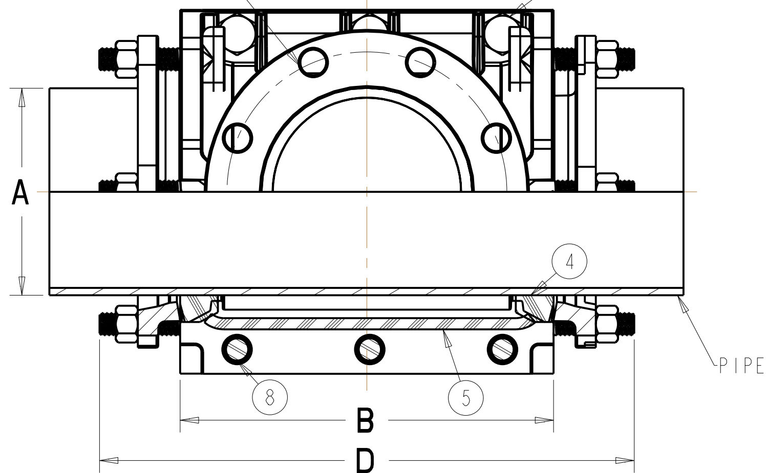
SECTION A-A
