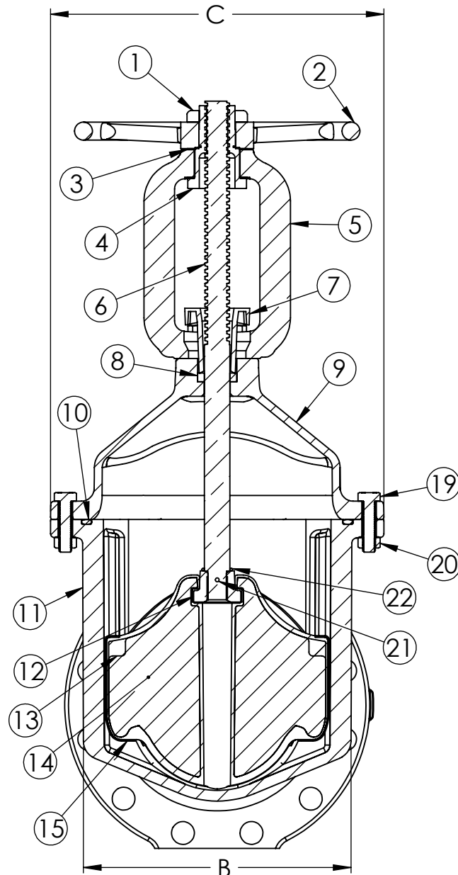
SECTION B-B SCALE 3 : 20
