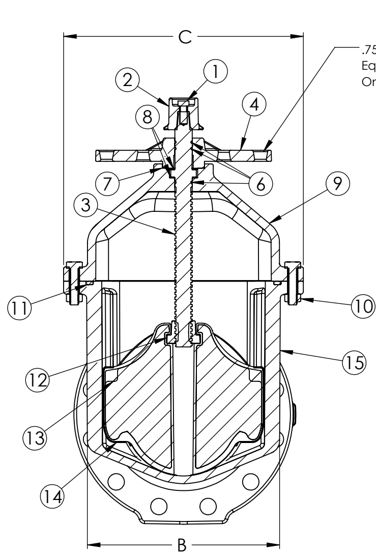
SECTION B-B SCALE 3 : 20
