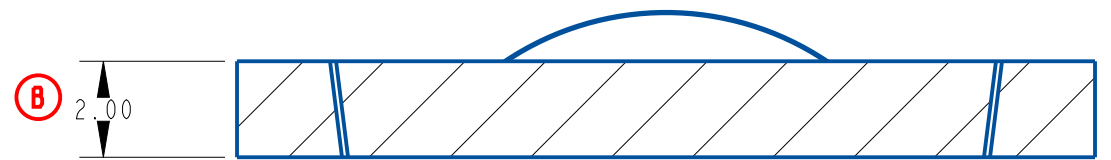
SECTION A-A
