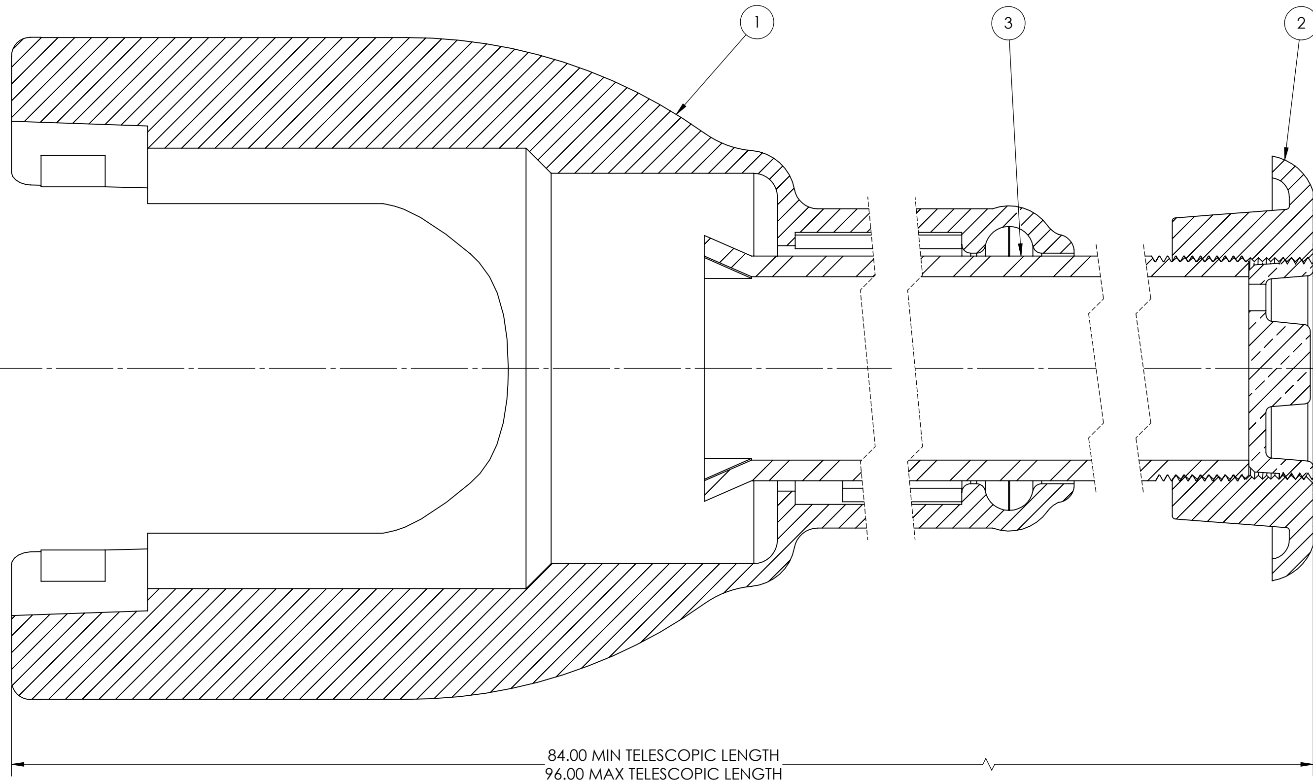
SECTION A-A
