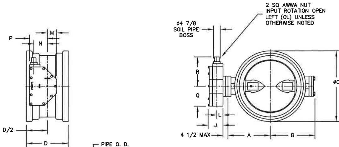
ACTUATOR POSITION 1
